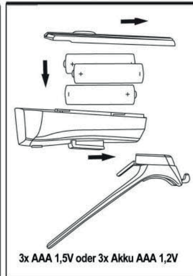
Batteriewechsel
